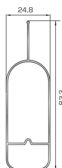
40525 W=46.4\text{gr/m} A=0.246\text{m}^2/\text{m}
