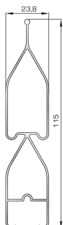
40415 W=79.4\text{gr/m} A=0.342\text{m}^2/\text{m}
