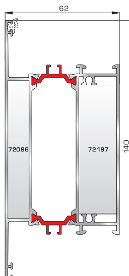
Frame muntin (Big)
